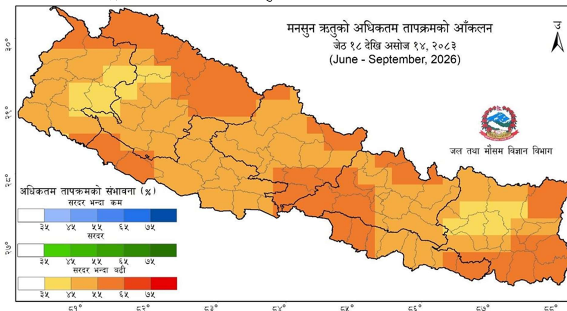
चित्र २: २०८३ को मनसुन ऋतुको अधिकतम तापक्रमको सर्वाधिक सम्भावना (highest probability) (%)
