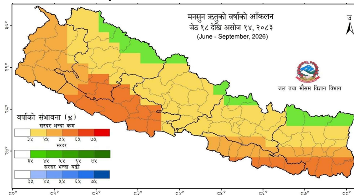
चित्र १: २०८३ को मनसुन ऋतुको वर्षाको सर्वाधिक सम्भावना (highest probability) (%)
