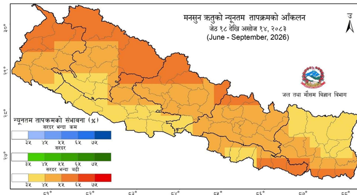
चित्र ३: २०८३ को मनसुन ऋतुको न्यूनतम तापक्रमको सर्वाधिक सम्भावना (highest probability) (%)
