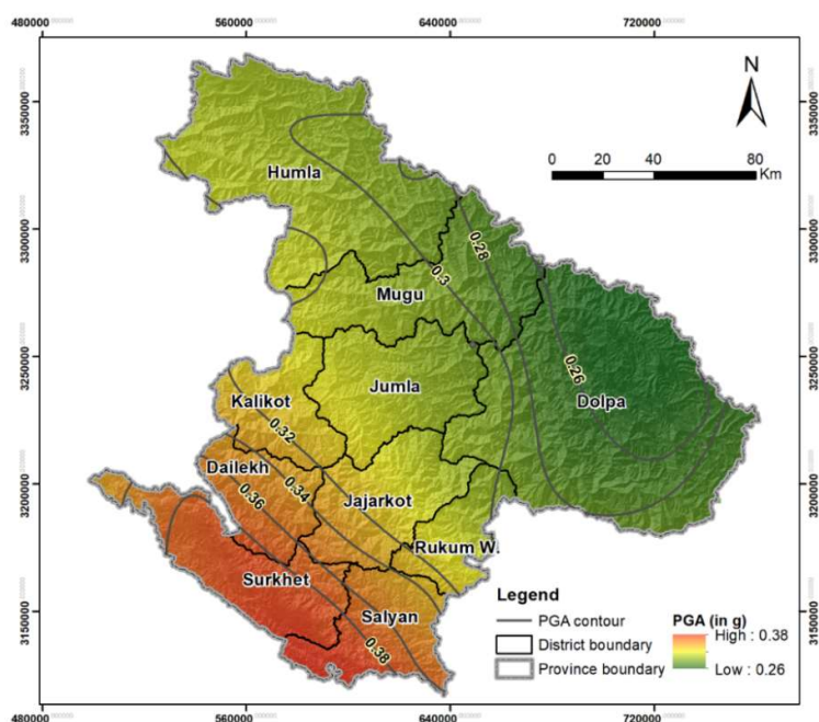
चित्र २: कर्णाली प्रदेशको भूकम्पीय जोखिम नक्शा
